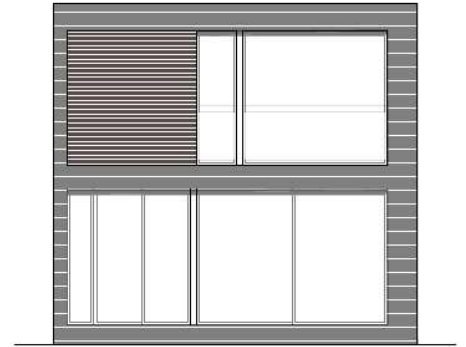
ALZADO TRASERO
