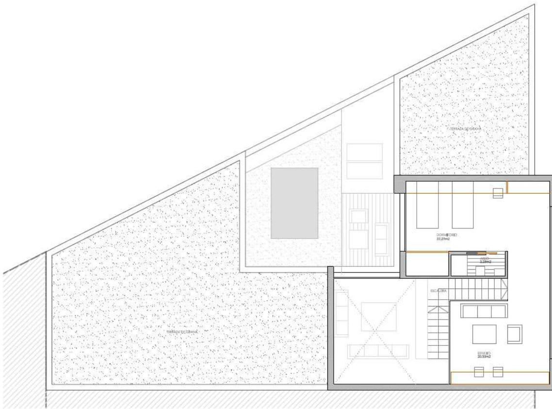
PLANTA PRIMERA/CUBIERTA
