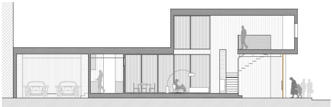
SECCION INTERIOR 2
