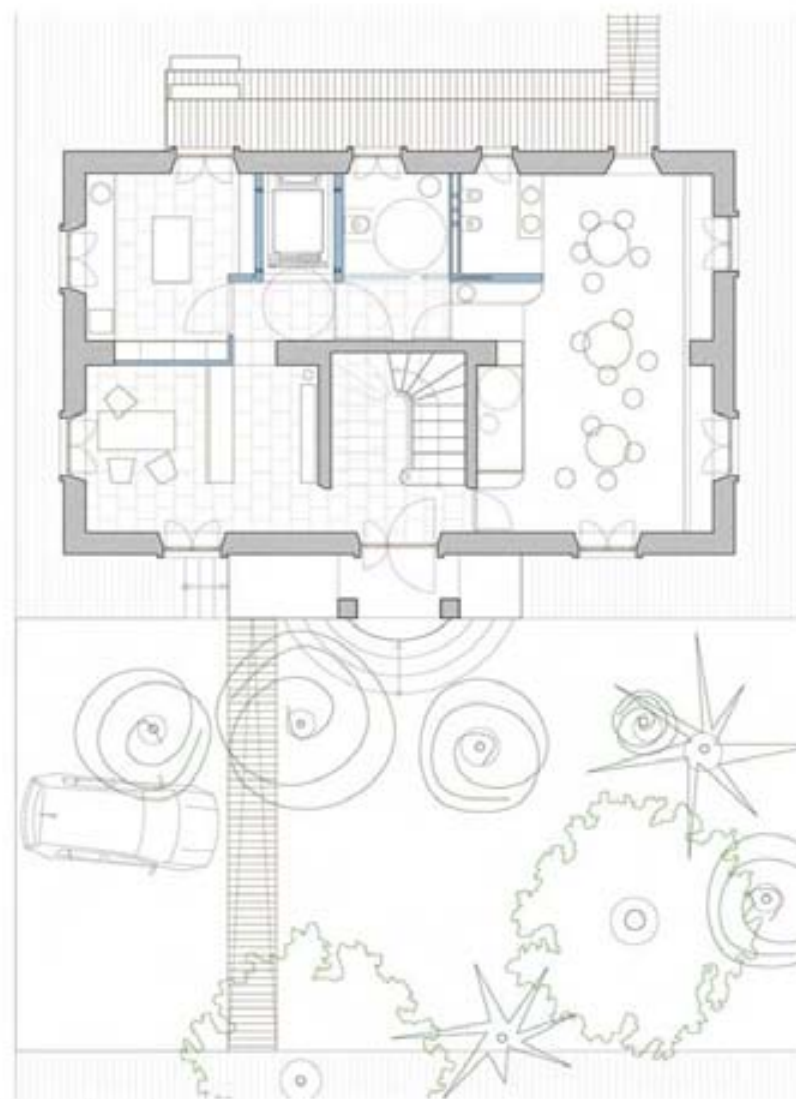
PLANTA BAJA, Propuesta Escala 1:100
