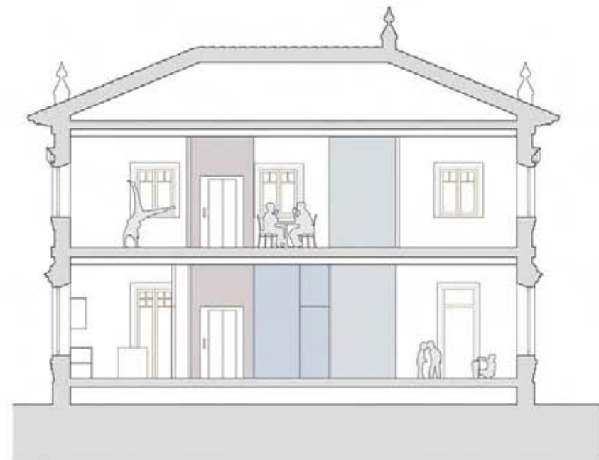
SECCIÓN LONGITUDINAL. Propuesta Escala 1:100
