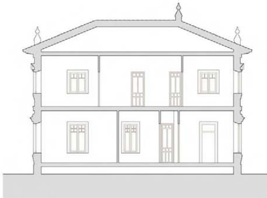
SECCIÓN LONGITUDINAL. Estado Actual Escala 1:100
