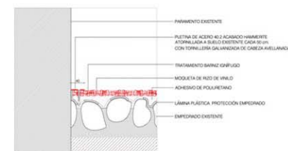
SV 1. ENCUENTRO ENTRE ALFOMBRA Y PARAMENTO VERTICAL
