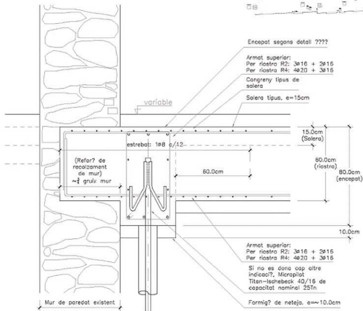
D-02. Secció tipus de encepats amb recolzament de mur i riostra
